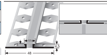
301 S \varnothing 3 mm geschlossen gestanzt, mit Silikonfuge
