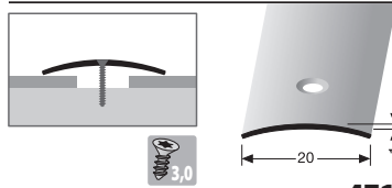
471 mittig versenkt gebohrt
