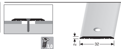
443 mittig versenkt gebohrt
