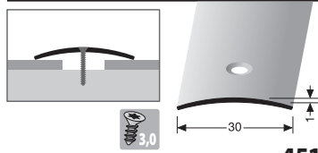
451 mittig versenkt gebohrt
