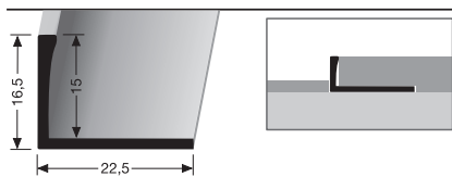
306 U \varnothing 15 mm ungestanzt
