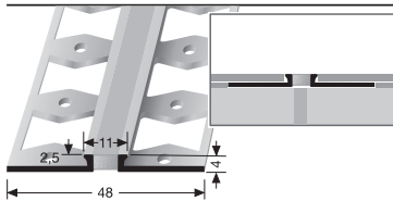
300 S \varnothing 2,5 mm geschlossen gestanzt, mit Silikonfuge
