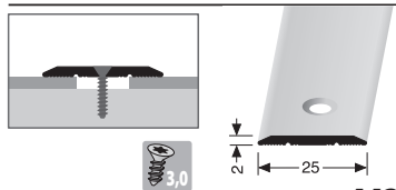
442 mittig versenkt gebohrt
